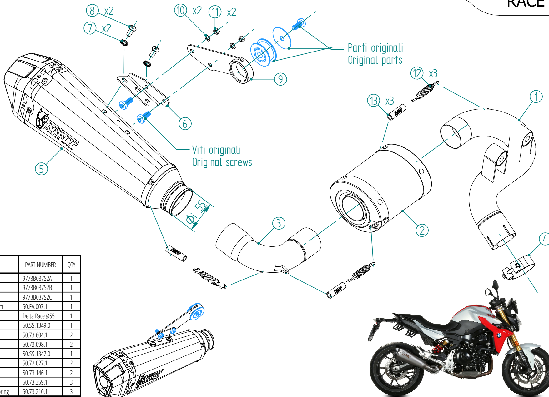
Impianto no kat - No kat pipe 00.73.B.037.C1
